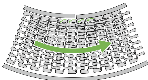
カーブコンベア
