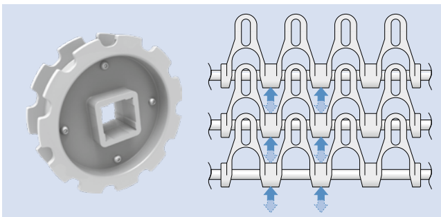
スプロケットの取り付け
