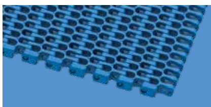
S18 | 開口率44% | ガイド付きグリッドト ップ 2.2
