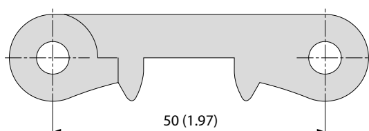
側面図 (比例1:1)
