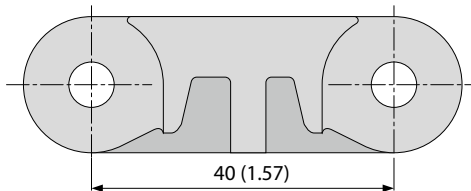
側面図 (比例1:1)
