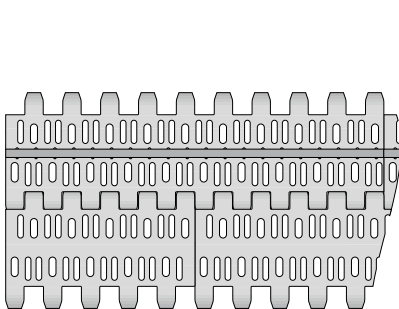
標準構成 S6.1-23 NCL PMU
