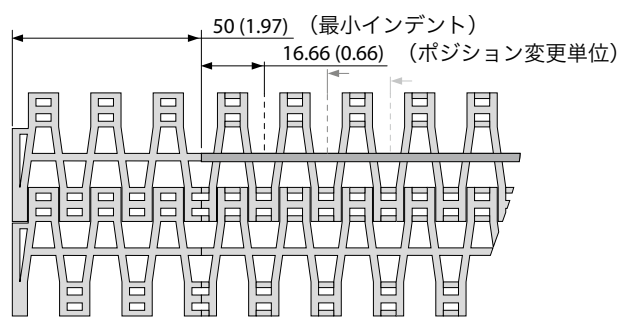
インデント付き構成 S2-57 GRT PMC
