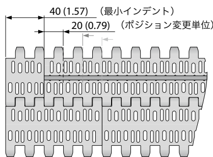
インデント付き構成 S6.1-23 NCL PMU
