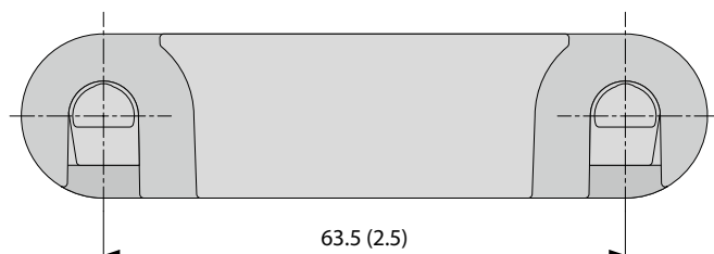
側面図 (比例1:1)
