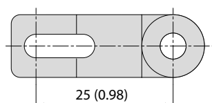
側面図 (比例1:1)
