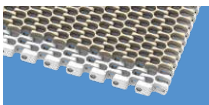
S18 | 開口率44% | フリックショントップ 1
