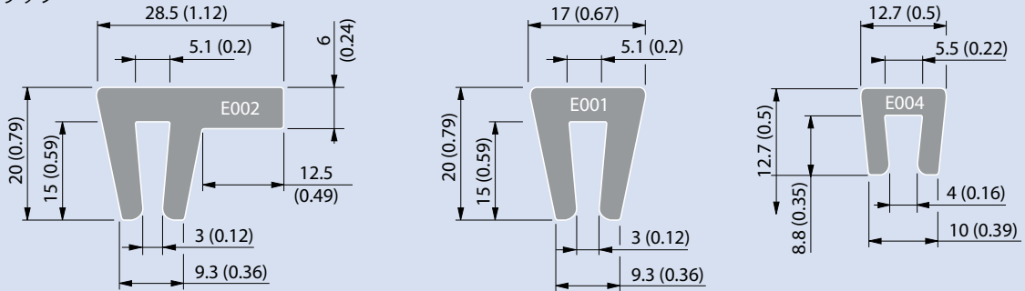
押出摩耗ストリップ
