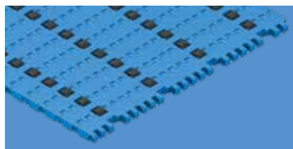
S8.1 | 開口率0% | PRR付FLT
