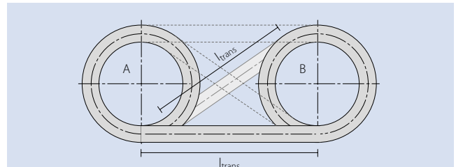
ダブルスパイラル
